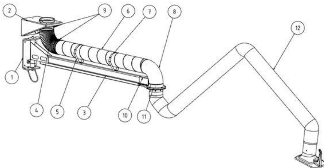
Abb. 2: Auslegerarm
