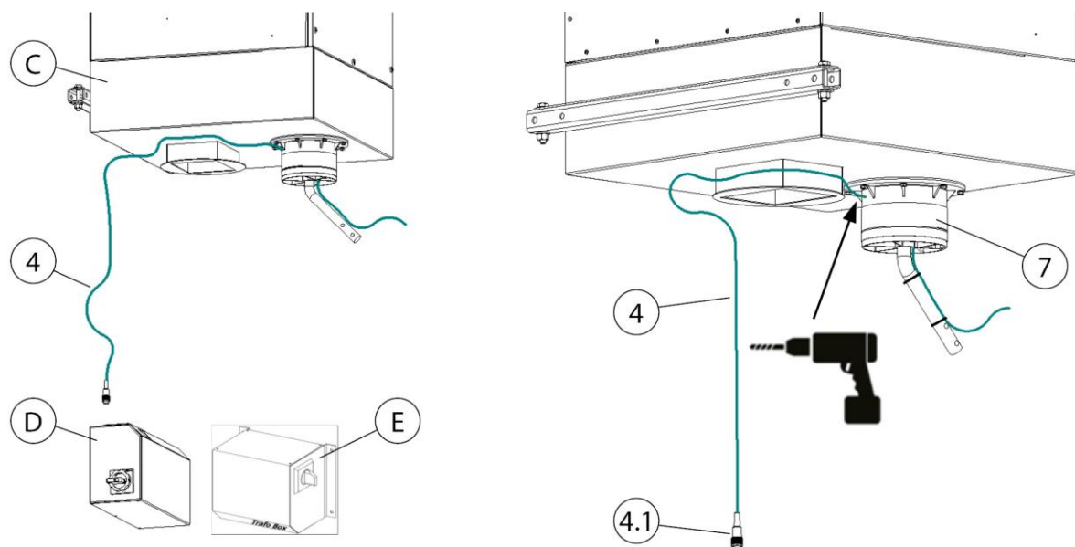
Abb. 14: Kabelverlegung – stationäres Gerät
