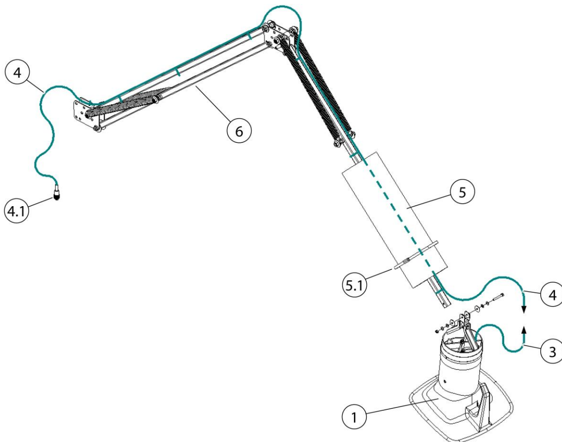
Abb. 13: Kabelverlegung - Absaugarm 2-4 Meter
