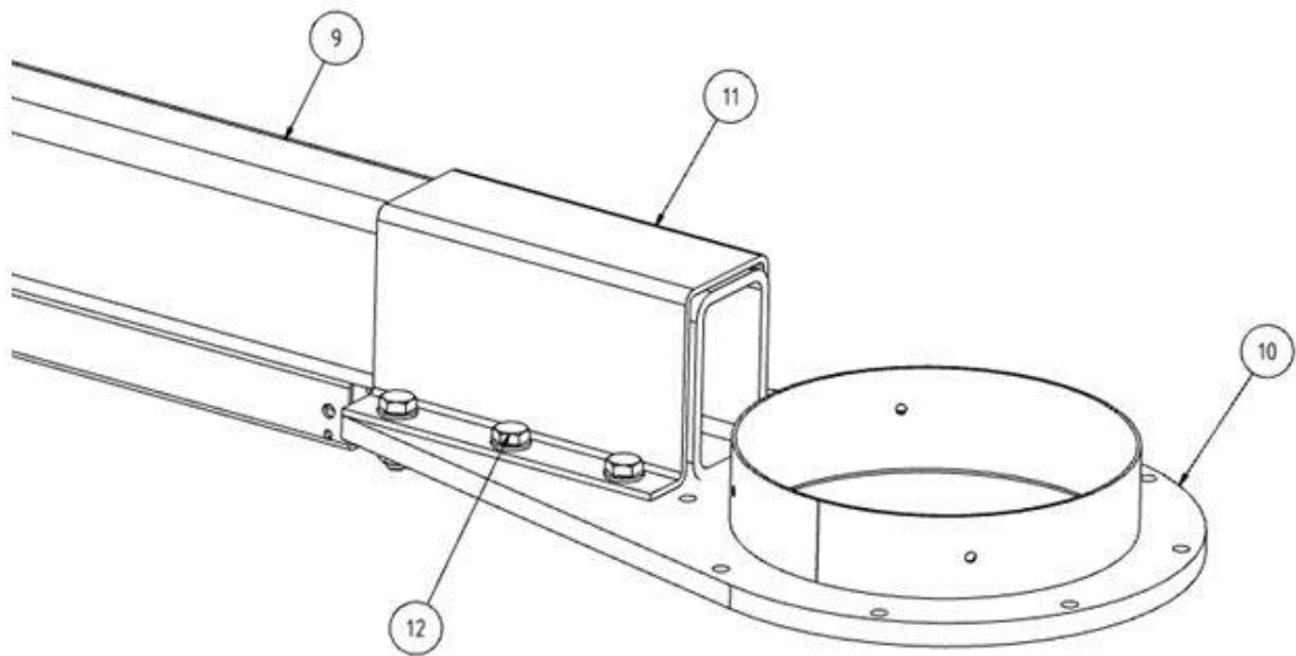
Abb. 6: Absaugarmhalterung
