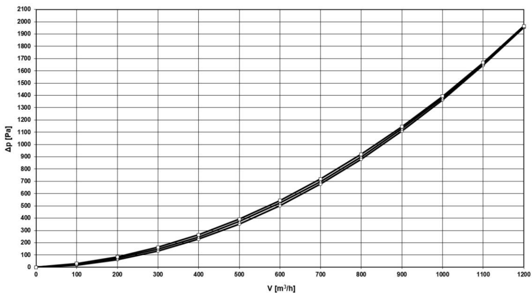
Abb. 16: Druckverlustdiagramm
